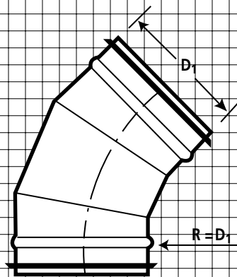
45° 3-PC. ELBOW E45T
